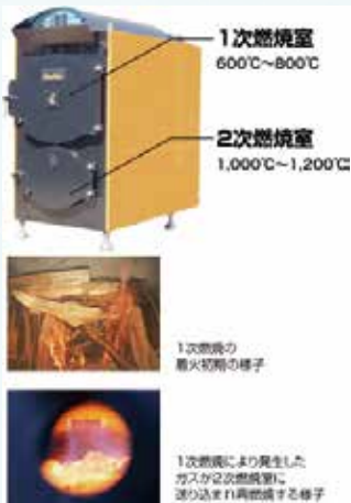
薪ボイラー
